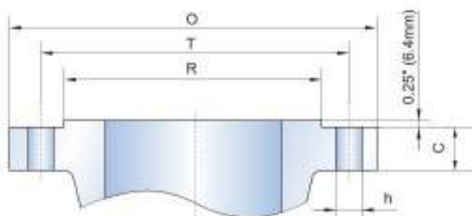
CLASS 600-2500 RF
